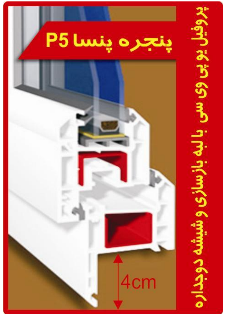
پروفیل باز سازی upvc
