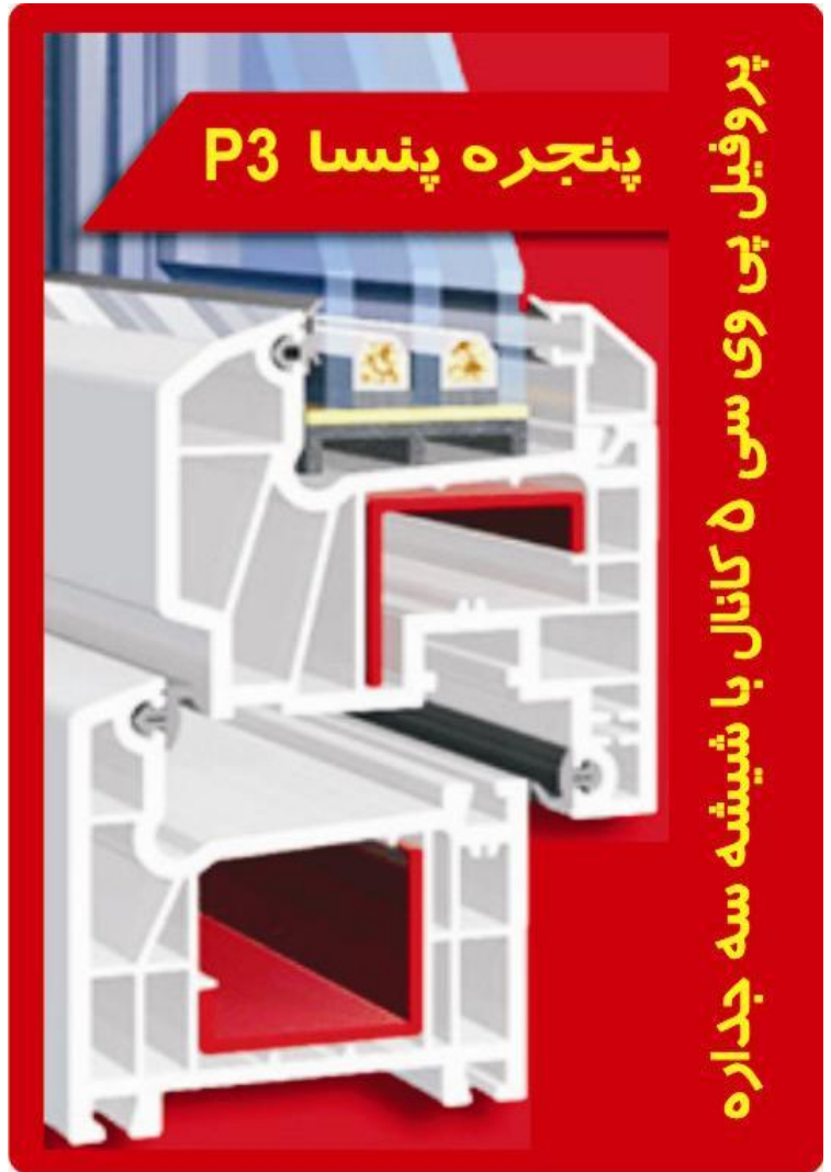
پروفیل پنج کانال upvc با شیشه سه جداره
